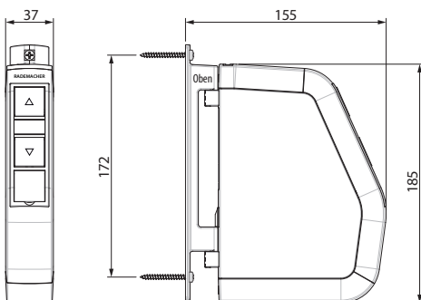
Abmessungen Schwenkwickler Standard DuoFern:
